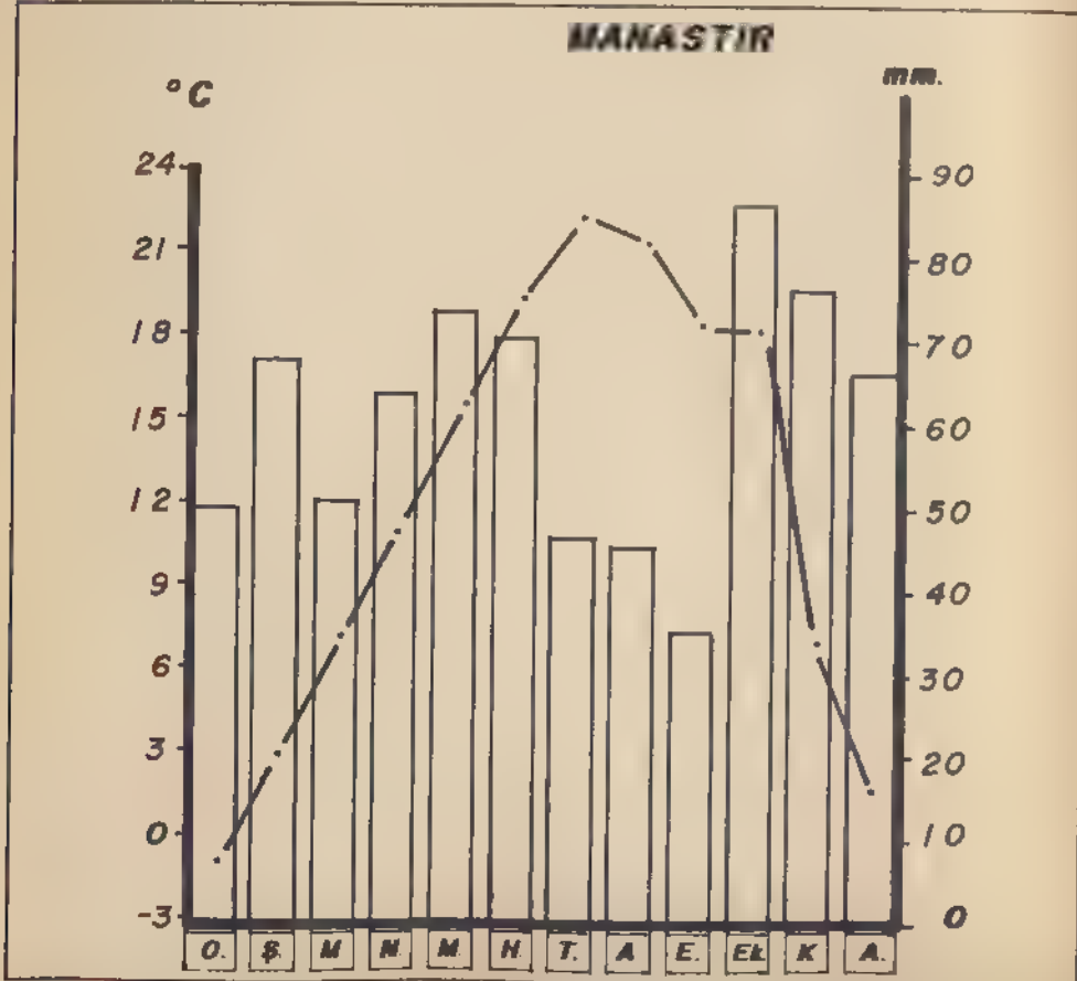
Şekil 14- Manastır'ın iklim diyagramı. Sıcaklık kesik çizgi ile, yağış sütunlarla gösterilmiştir.
